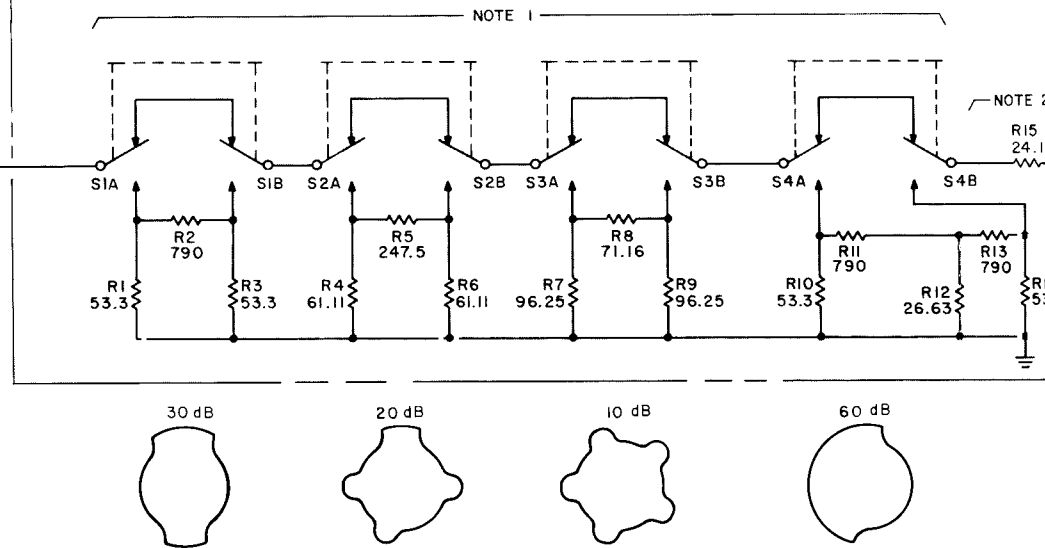
A7 ATTENUATOR ASSY (08601-6007)
