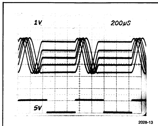
2-15図 位相調整。トリガ・モードでのPHASEダイヤルによる動作を示しています。5個の重ねられた波形は位相調整による結果です。このダイヤルにより \pm 80^\circ の位相を変えられます。下側の波形はトリガ信号です。
