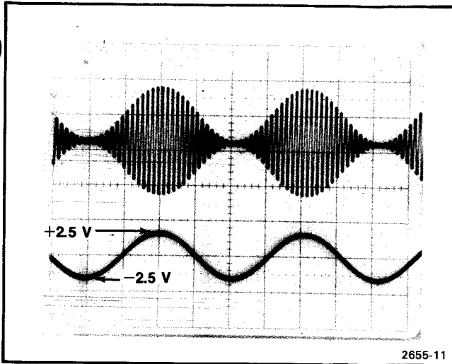
2-17図 振幅変調。上側の波形は100%変調のエンベロープをまし、下側は変調信号を示しています。±2.5Vで出力を100%変調しています(0Vを中心に5V p-p)。
