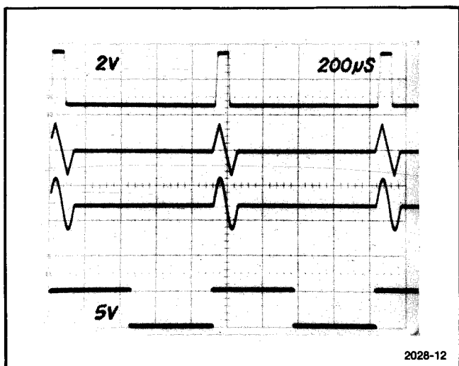
2-14図 トリガ動作。TRIGモードが選択され、トリガINPUTコネクタにトリガ信号が入力された時の、上側3個が出力波形で、下側がトリガ波形です。出力波形が1周期であることを注意して下さい。
