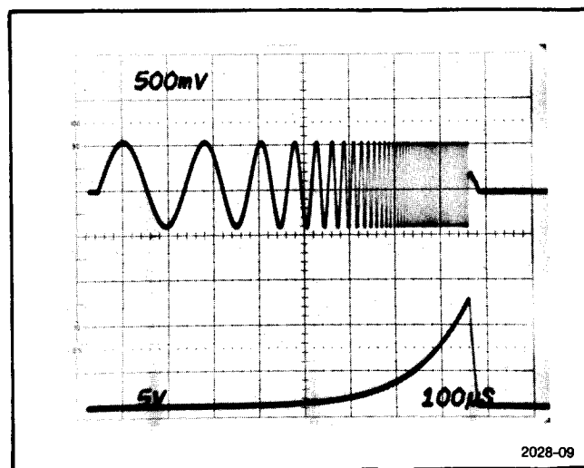
Fig. 2-11. BALAYAGE LOGARITHMIQUE. Procéder de manière identique que pour la figure 2-10. Sélectionner la rampe logarithmique. La fréquence est modulée de façon logarithmique. La tension de la rampe logarithmique n'est pas disponible extérieurement.
