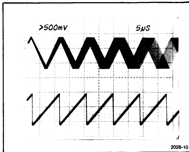
Fig. 2-12. BALAYAGE A BANDE ETROITE. La trace supérieure illustre un signal triangulaire balayé par une rampe linéaire. La fréquence de départ est de 9,52 kHz et la fréquence d'arrêt est de 10,52 kHz. Cette fonction est utile pour des tests par balayage à bande étroite. La trace inférieure correspond à la rampe de balayage.
