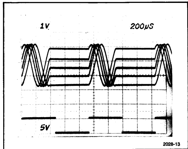
Abb. 2-15. PHASENGESTEUERTER BETRIEB. Das Bild zeigt die Funktion des Phaseeinstellers bei getriggertem Betrieb. Die fünf überlagerten Strahle zeigen die Wirkung des Phaseeinstellers. Dieser Einsteller bietet ca. \pm 80^\circ Phasenänderung. Das untere Signal ist das Triggersignal.
