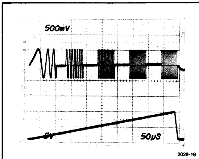
Abb. 2-21. TONFREQUENZBURST-TEST. Der untere Ablenkstrahl ist der lineare Sägezahn von dem Ausgang LIN SWEEP OUTPUT.
