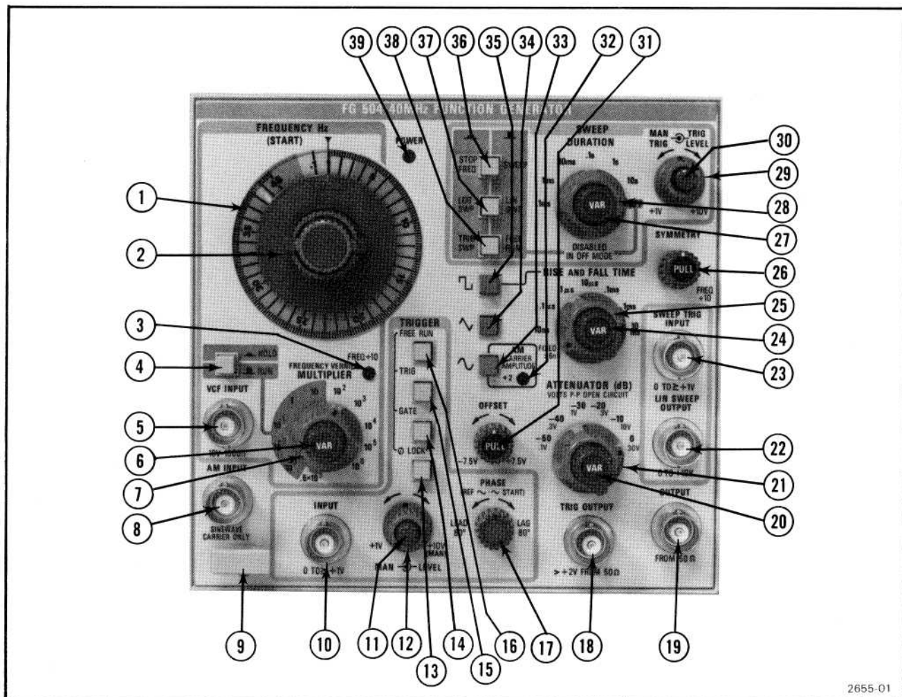
Abb. 2-2. Bedienungselemente und Anschlüsse der Frontplatte
