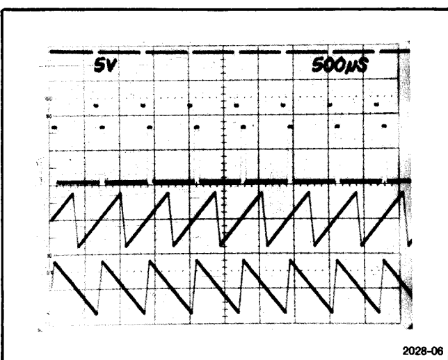
2-8図 のこぎり波とパルス。SYMMETRYコントロールを使ってこのような波形をつくることができます。
