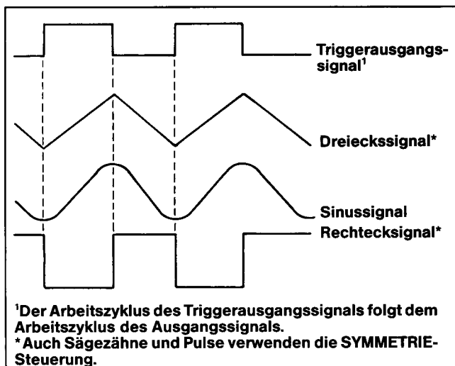
Abb. 2-6 Phasenbezug zwischen Ausgangssignalen und Triggerausgangssignal.
