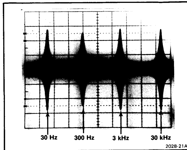
Fig. 2-23. Balayage logarithmique montrant un espacement régulier des fréquences de résonance du filtre.
