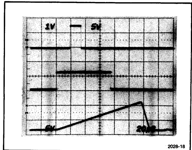
2-20図 遅延動作。遅延ゼネレータとして内部掃引ゼネレータを使用することにより広範囲な遅延時間が設定できます。中段はSWEEP TRIG INPUTに入力された基準信号波形です。下側の波形はLIN SWP OUTコネクタからのこぎり波です。このこぎり波を外トリガ入力コネクタに入力します。上側の波形は遅延出力パルスです。遅延時間は掃引時間幅と TRIG LEVELコントロールの設定に比例します。掃引を遅延ゼネレータとして使用する際はSTOP FREQダイヤルを左回し一杯になっていることを確認して下さい。
