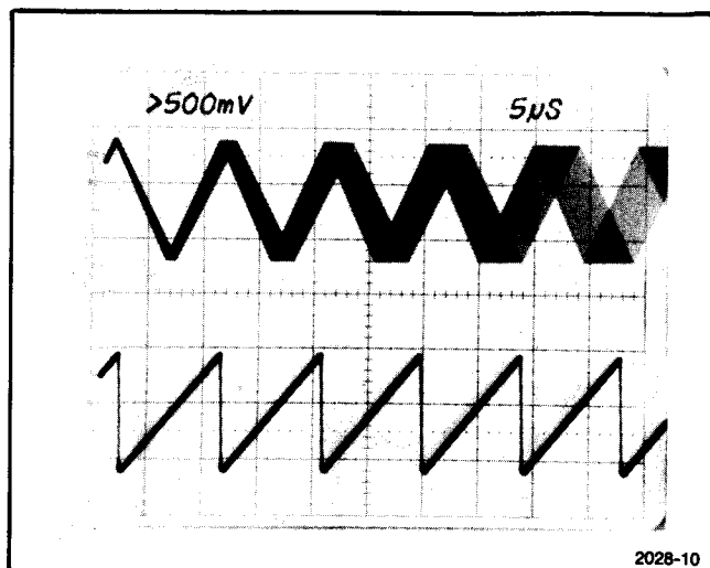
2-12図 狭い範囲の掃引。上側はスタート周波数が9.52kHz、ストップ周波数が10.52kHzのリニア掃引による三角波です。これは狭い帯域での掃引試験を行う時に有効です。下側の波形は掃引用のこぎり波です。
